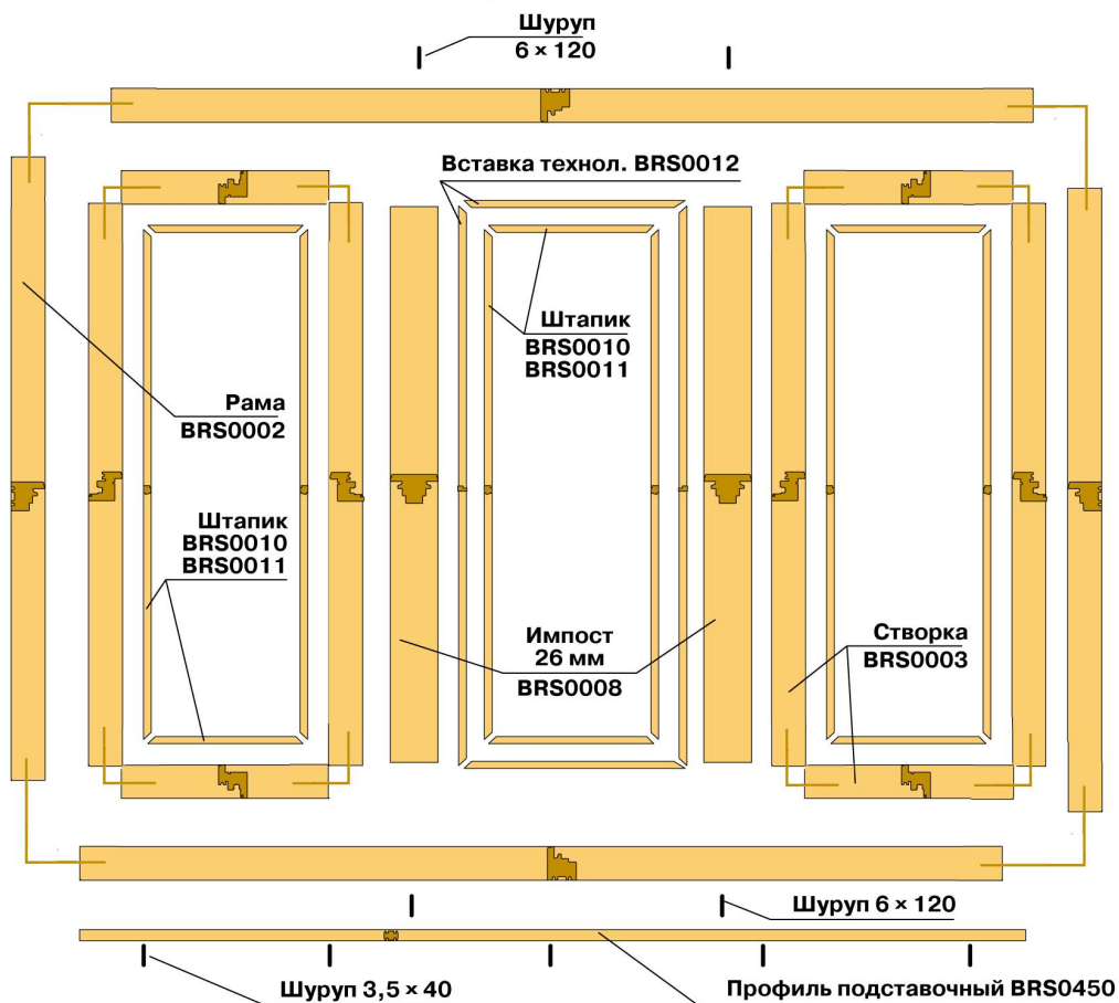
Комплектация трехстворчатого окна с глухой средней частью
